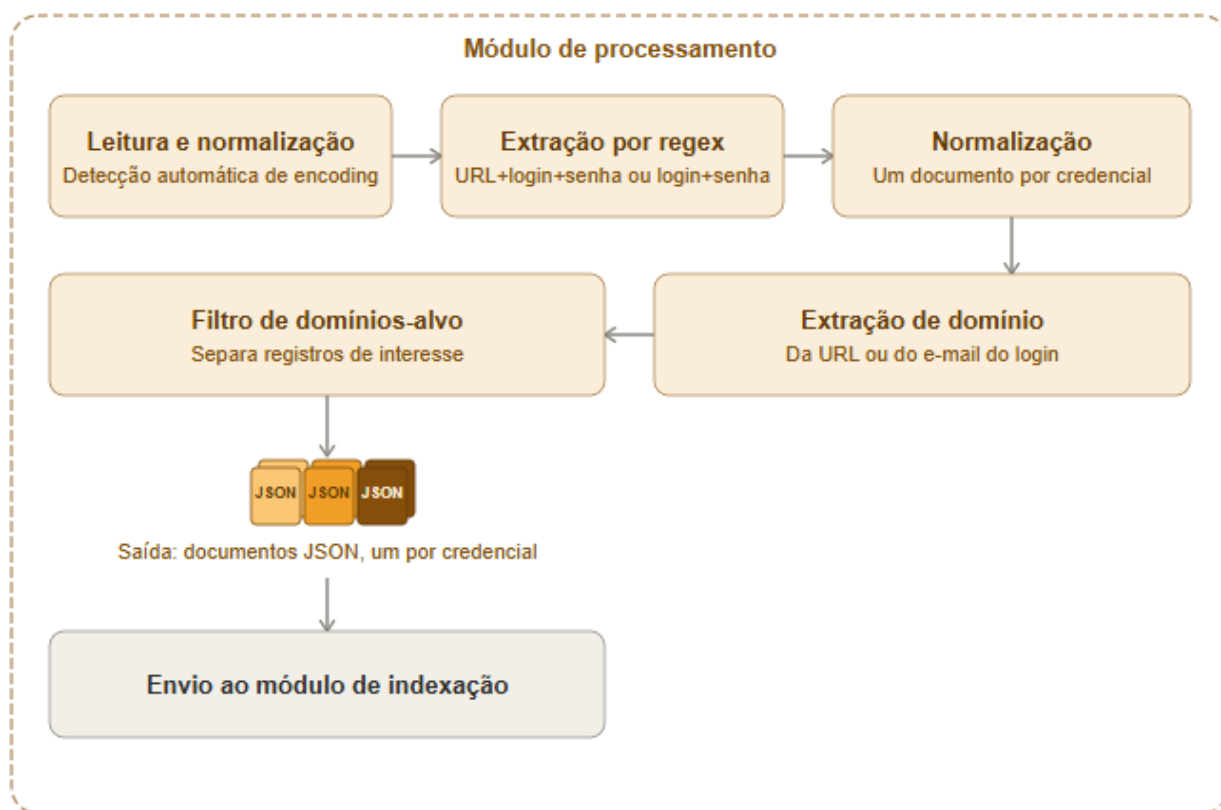
Figura 4.2: Fluxo de execução do módulo de processamento proposta nesta pesquisa.
