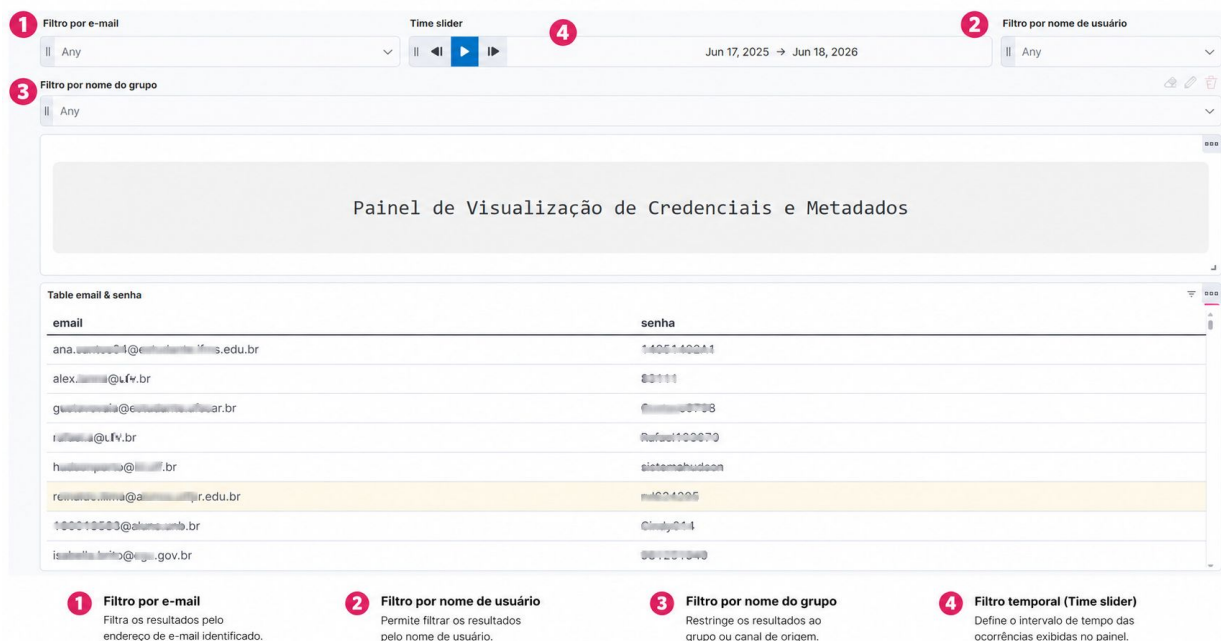
Figura 4.5: Mecanismos de filtragem implementados no painel analítico. (1) filtro por endereço de e-mail; (2) filtro por nome de usuário; (3) filtro por grupo monitorado; (4) filtro temporal.
