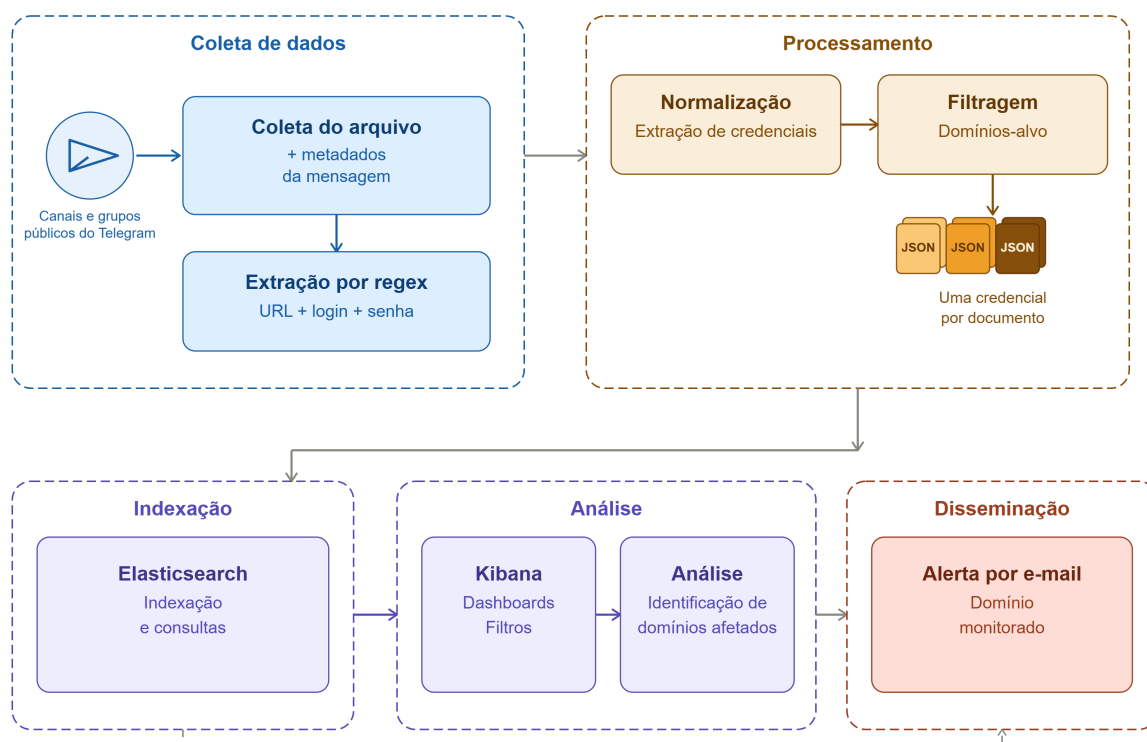
Figura 3.2: Arquitetura da pipeline proposta nesta pesquisa.
