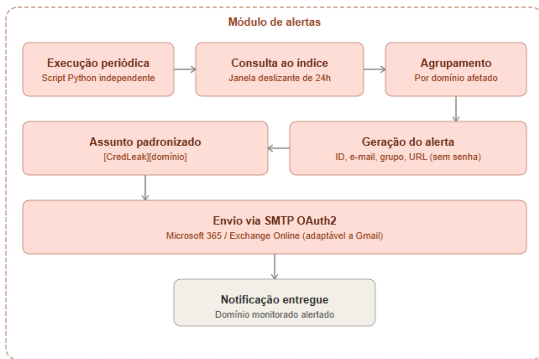
Figura 4.9: Fluxo de execução do módulo de alerta proposta nesta pesquisa.
