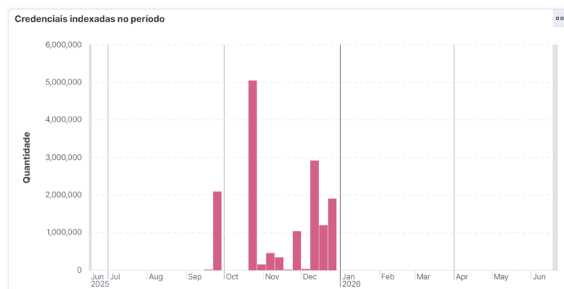
Figura 4.6: Distribuição temporal das credenciais indexadas durante a execução da prova de conceito.
