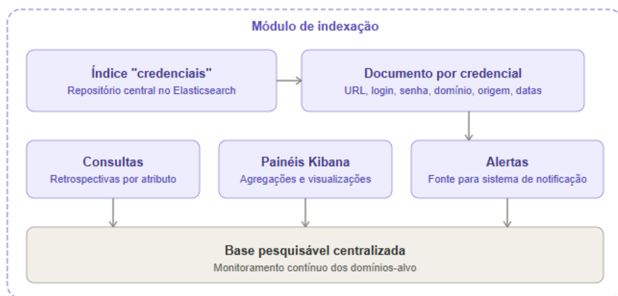
Figura 4.3: Fluxo de execução do módulo de indexação proposta nesta pesquisa.
