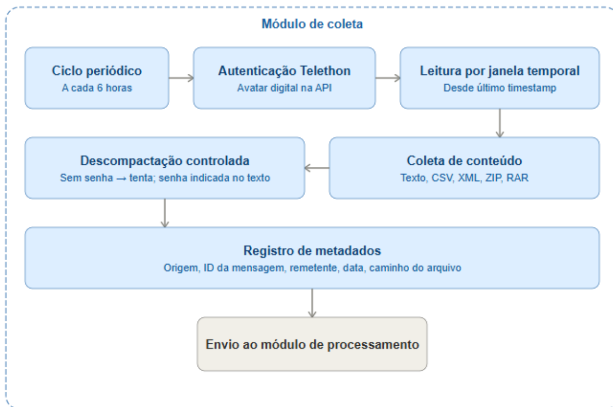
Figura 4.1: Fluxo de execução do módulo de coleta. proposta nesta pesquisa.
